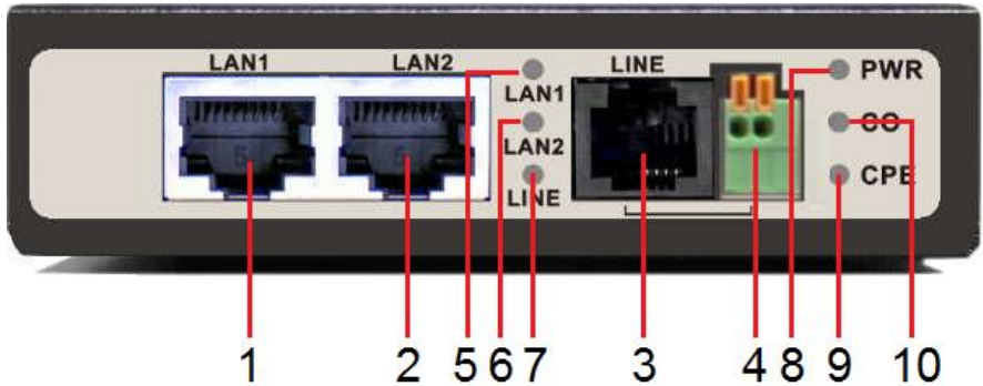
Рис. 2 Элементы передней панели TR-IP2.
